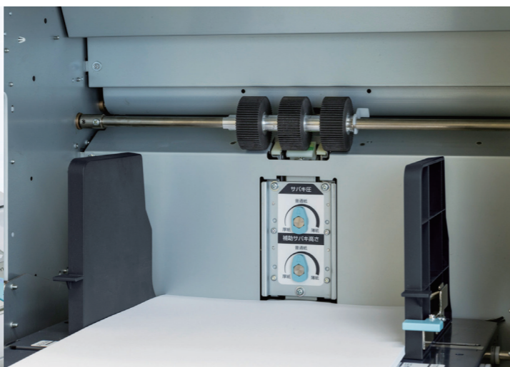
Rouleaux d'alimentation
